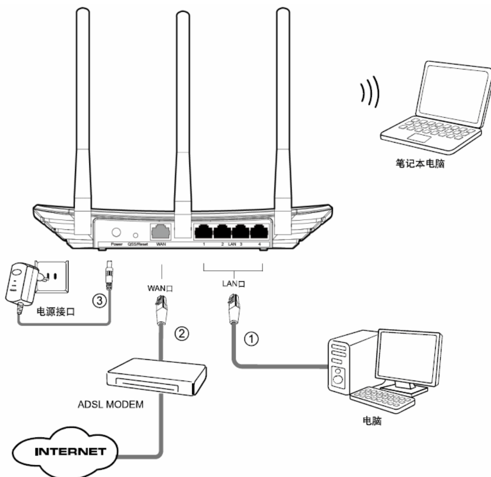
图 4-1 TL-WR880N 硬件安装示意图
