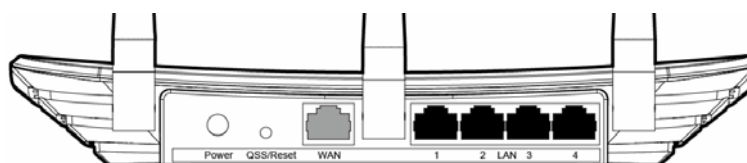
图 3-2 TL-WR880N 后面板示意图
